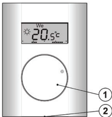
Abbildung 1: 1 – Drehregler mit Taste; 2 – Abdeckungsglasche
