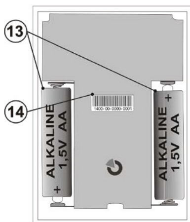
Abbildung 4: 13 – Batteriehalterungen; 14 – Seriennummer
